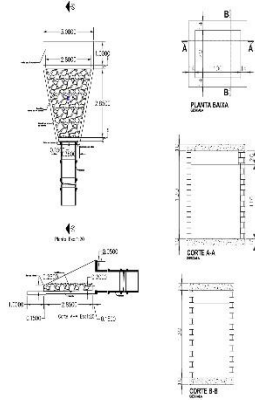
DETALHE BOCA DE LOBO
